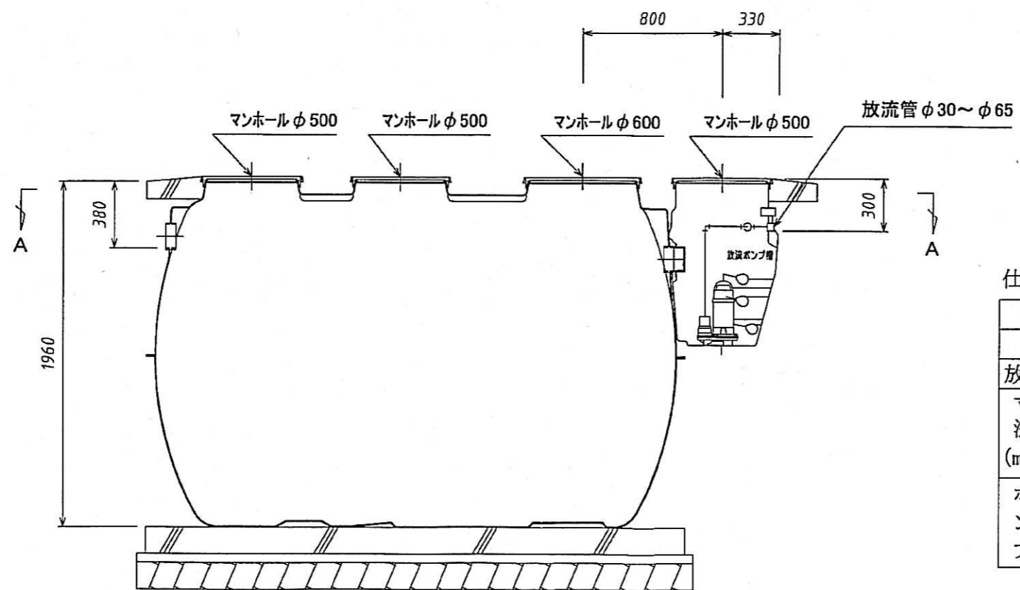
B-B断面図
