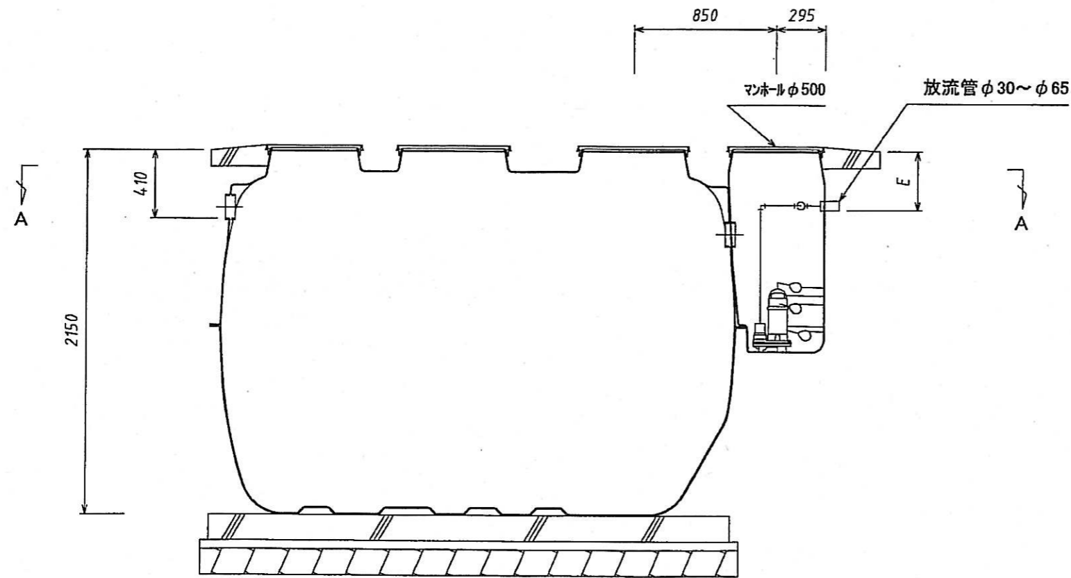
B-B断面図
