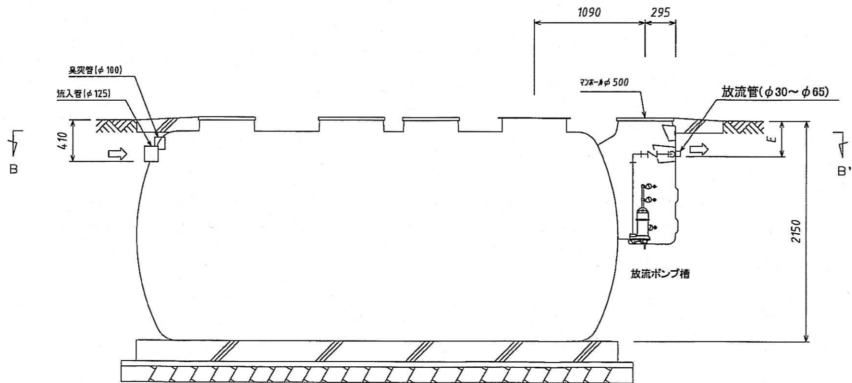
A-A' 断面図
