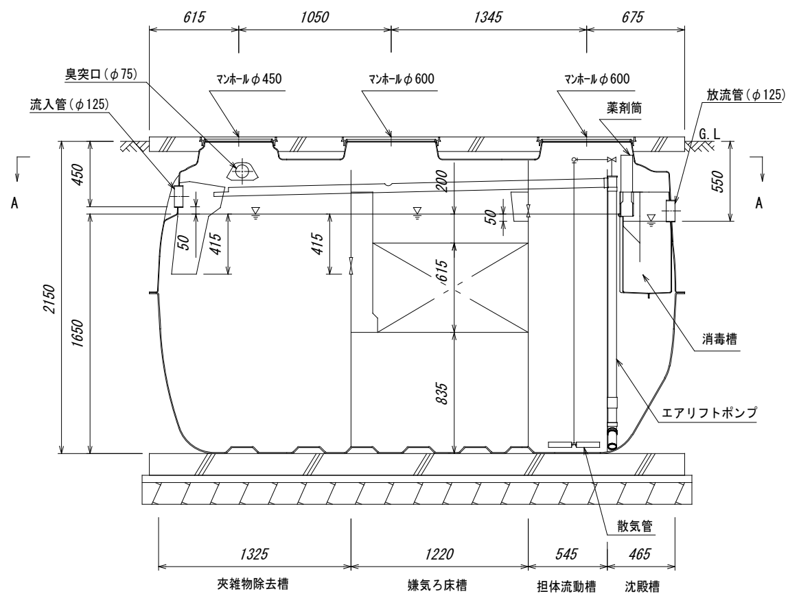
B-B断面図
