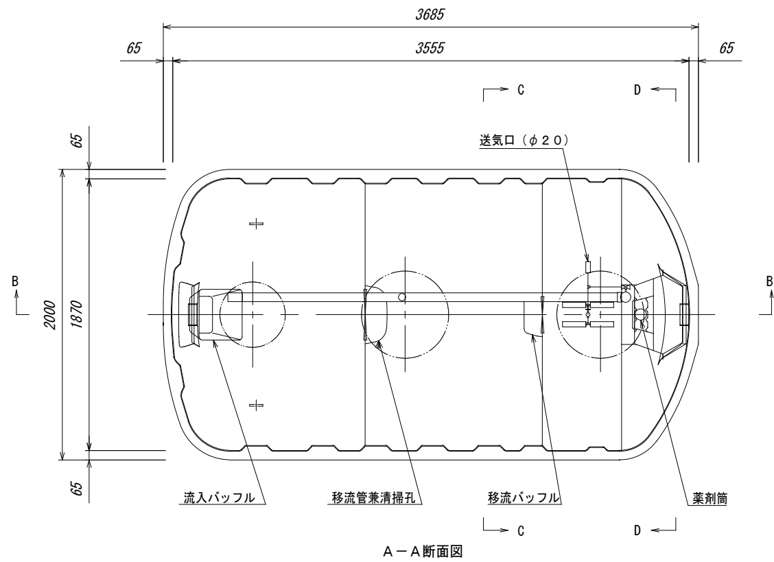
A-A断面図
