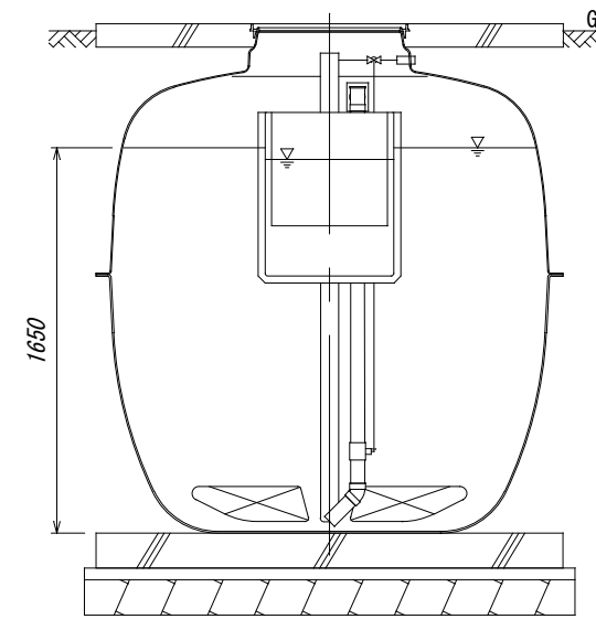
D-D断面図
